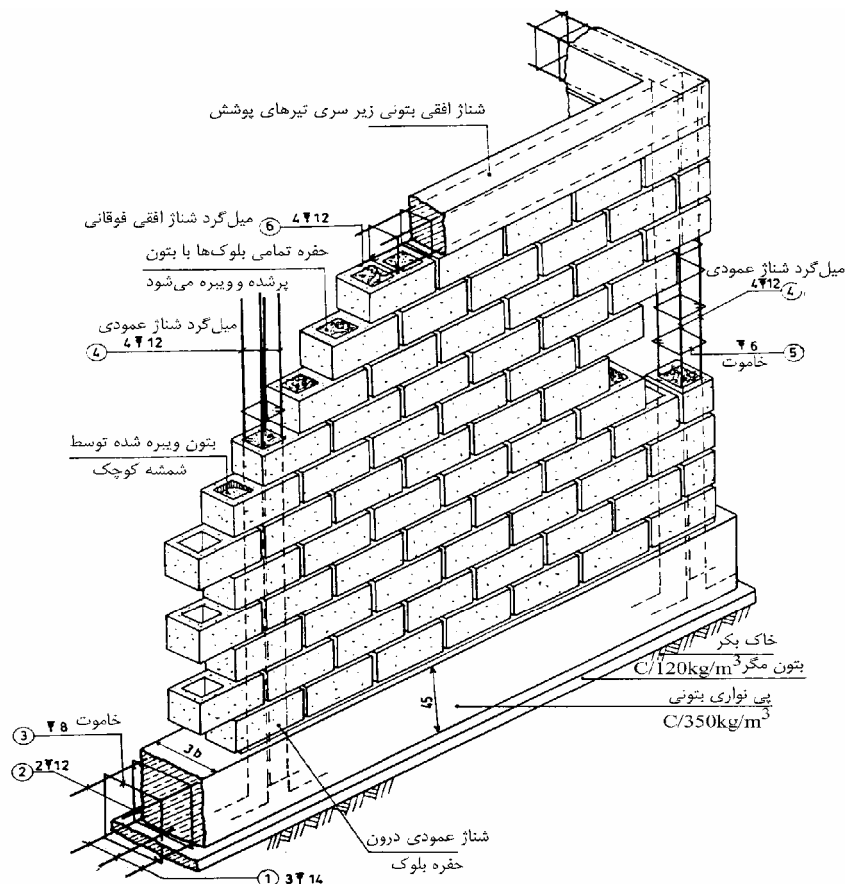
شکل ۸ جزئیات دیوار باربر بلوک سیمانی با کلاف‌بندی شناژهای عمود و افقی
