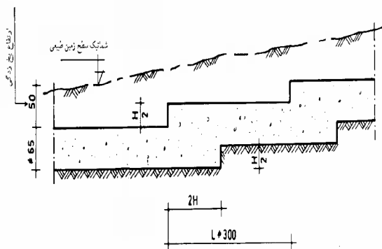
شکل ۱ پی سازی پله ای در زمین شیب دار
